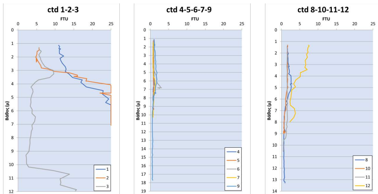
Εικόνα 5: Κατακόρυφες καταγραφές της θολερότητας (σε FTU) στην περιοχή του έργου της Μαρίνας Βουλιαγμένης κατά τη διάρκεια της 15 ης Ιουλίου 2021. Για τις θέσεις των μετρήσεων βλέπε την Εικόνα 3.
