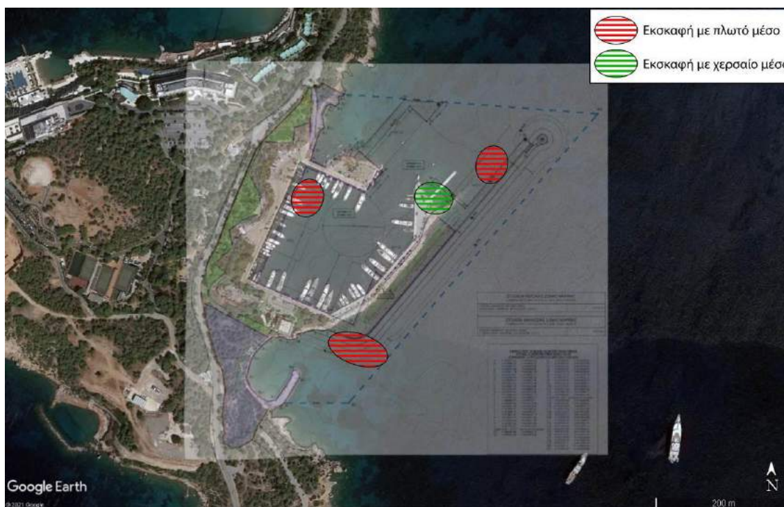
Εικόνα 4: Ενεργές εκσκαφές/βυθοκορήσεις στην περιοχή των έργων της Μαρίνας Βουλιαγμένης κατά τη διάρκεια της 15 ης Ιουλίου 2021.
