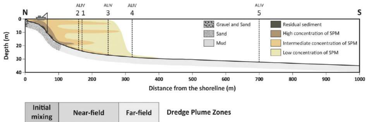
Εικόνα 1: Ζώνες διάχυσης του νέφους των επαναιωρημένων στερεών υλικών που προέκυψε από εντατική βυθοκόρηση στη περιοχή του Αλιβερίου, Νότιος Ευβοϊκός Κόλπος (Kanellopoulos et al. 2020).
