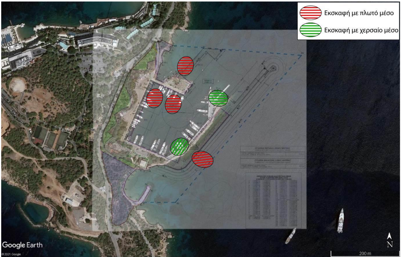
Εικόνα 1: Οριζοντιογραφία του έργου με τις εργασίες βυθοκόρησης.
