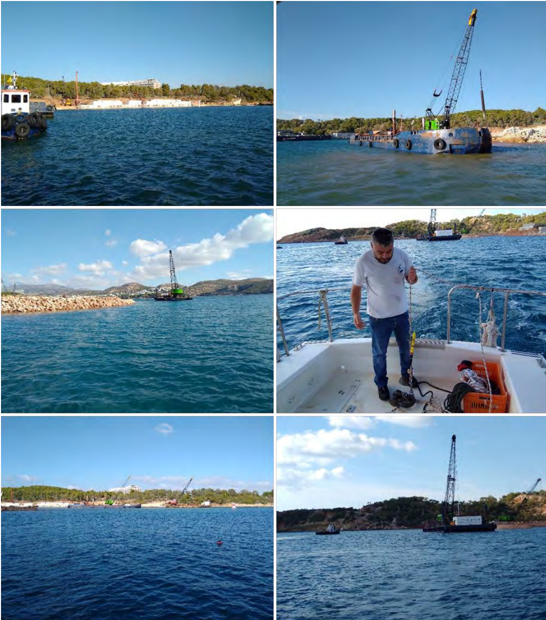
Εικόνα 2: Εργασίες πεδίου με νεφελόμετρο, το οποίο χρησιμοποιήθηκε για τη συλλογή μετρήσεων στην περιοχή του έργου της Μαρίνας Βουλιαγμένης την 27 η Οκτωβρίου 2021
