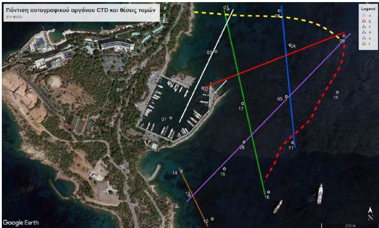
Εικόνα 3: Θέσεις μέτρησης της θολερότητας στην περιοχή του έργου της Μαρίνας Βουλιαγμένης κατά τη διάρκεια της 27 ης Οκτωβρίου 2021. Η άσπρη, η κόκκινη, η πράσινη η μπλε και η μωβ γραμμή αντιπροσωπεύουν τις γεωγραφικές θέσεις των τομών των Εικόνων 6α, 6β, 6γ, 6δ 6ε και 6στ αντίστοιχα. Με κίτρινη και κόκκινη σιτική γραμμή αποτυπώνονται οι θέσεις πόντισης των κουρτινών υλούς.
