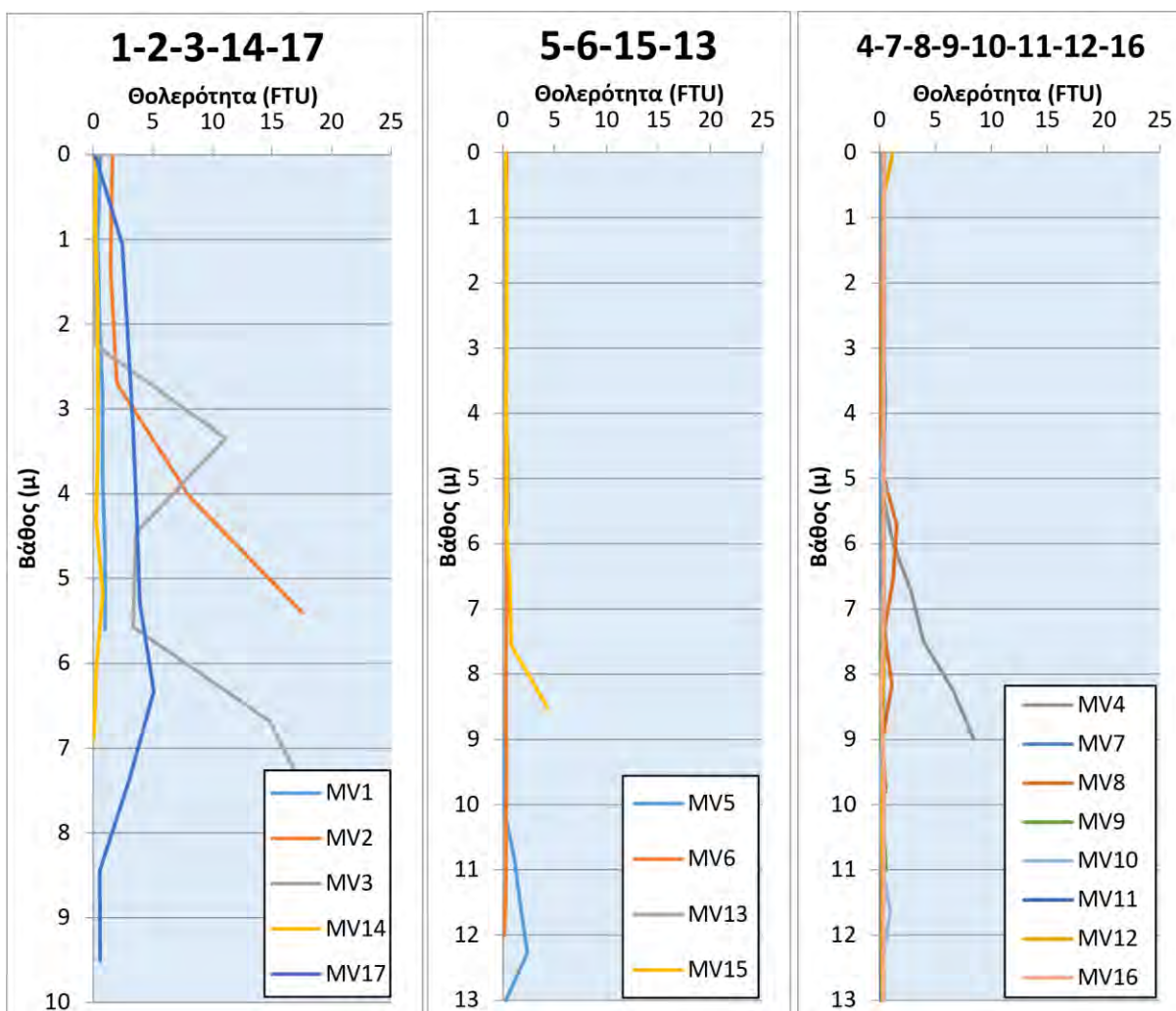
Εικόνα 5: Κατακόρυφες καταγραφές της θολερότητας (σε FTU) στην περιοχή του έργου της Μαρίνας Βουλιαγμένης κατά τη διάρκεια της 27 ης Οκτωβρίου 2021. Για τις θέσεις των μετρήσεων βλέπε Εικόνα 3.
