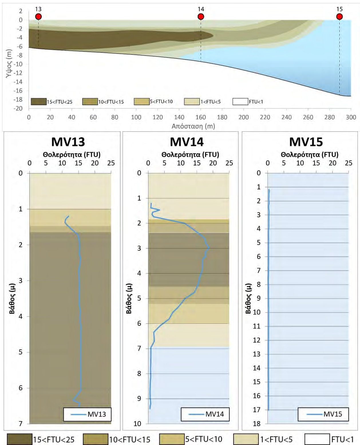
Εικόνα 6: Σχηματική αναπαράσταση της διασποράς/διάχυσης του παραγόμενου νεφελώματος από τις εργασίες εκσκαφής/βυθοκόρησης της 11 ης Αυγούστου 2021. Για τις θέσεις των μετρήσεων βλέπε την Εικόνα 3 .
