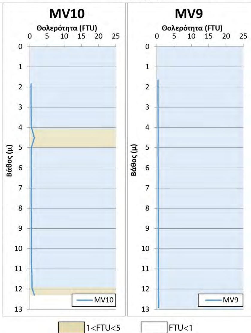
Εικόνα 6: Σχηματική αναπαράσταση της διασποράς/διάχυσης του παραγόμενου νεφελώματος από τις εργασίες εκσκαφής/βυθοκόρησης της 14 ης Σεπτεμβρίου. Για τις θέσεις των μετρήσεων βλέπε την Εικόνα 3.
