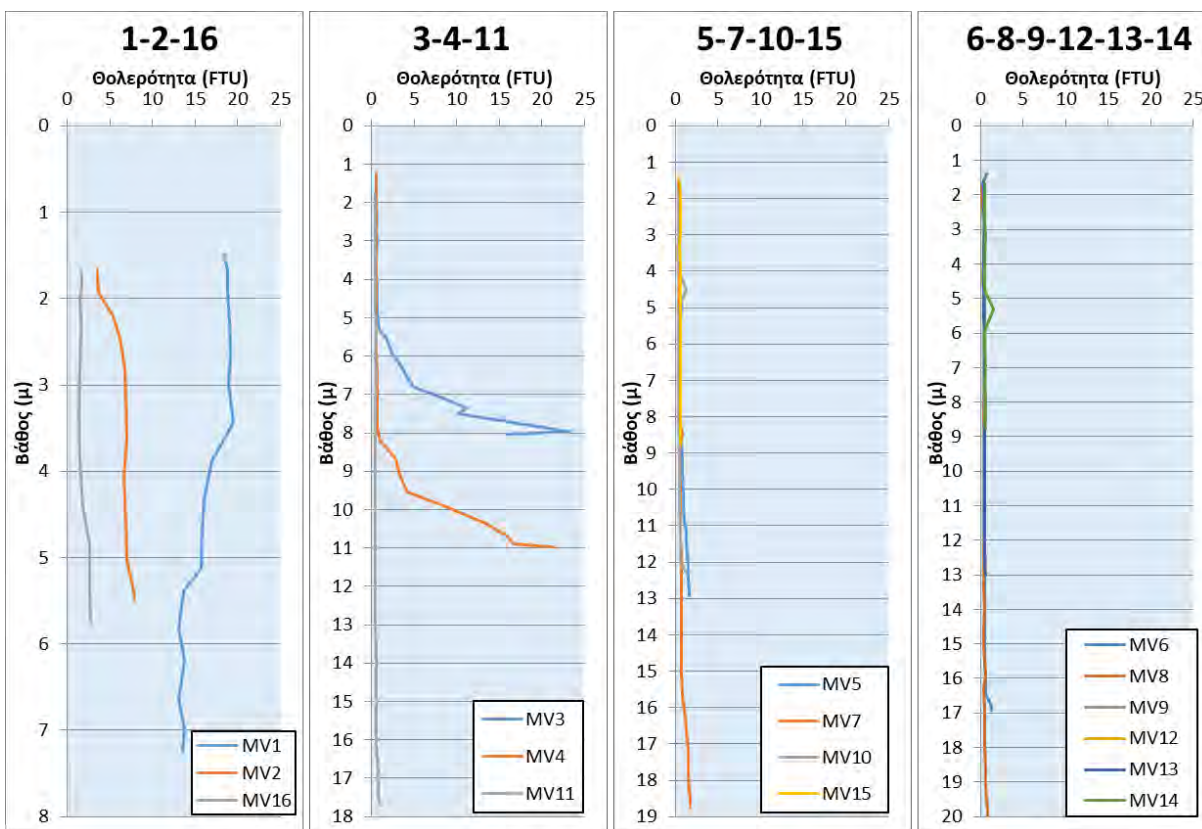
Εικόνα 5: Κατακόρυφες καταγραφές της θολερότητας (σε FTU) στην περιοχή του έργου της Μαρίνας Βουλιαγμένης κατά τη διάρκεια της 14 ης Σεπτεμβρίου 2021. Για τις θέσεις των μετρήσεων βλέπε Εικόνα 3.
