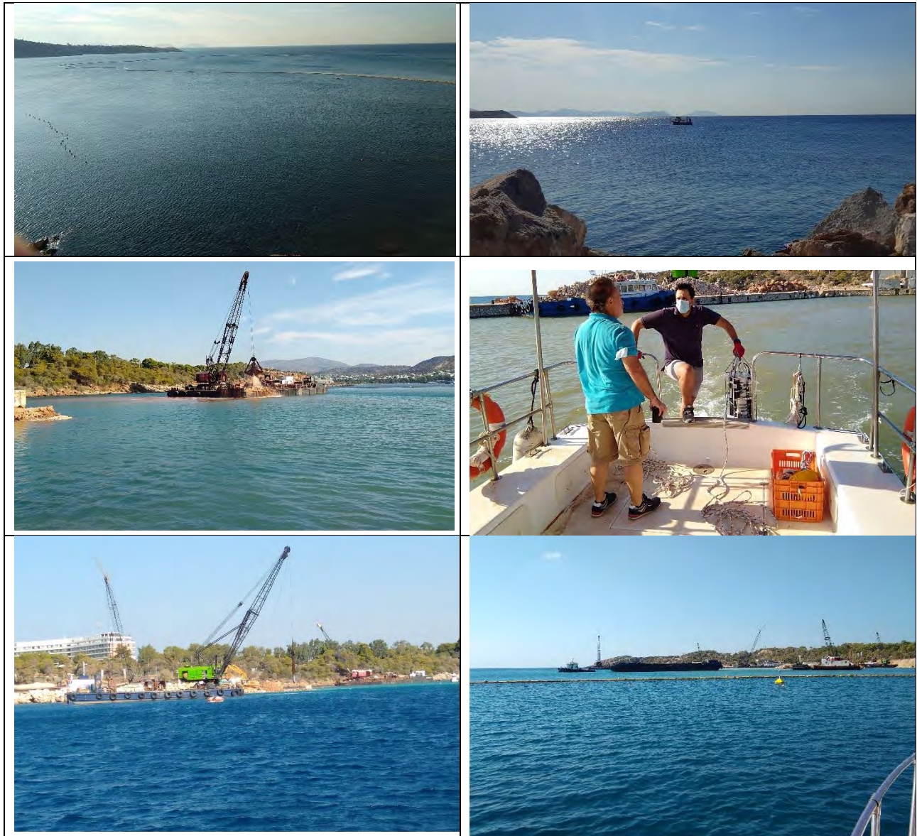
Εικόνα 2: Εργασίες πεδίου με νεφελόμετρο προσαρμοσμένο σε αυτογραφικό σύστημα CTD, το οποίο χρησιμοποιήθηκε για τη συλλογή μετρήσεων στην περιοχή του έργου της Μαρίνας Βουλιαγμένης την 14 η Σεπτεμβρίου 2021
