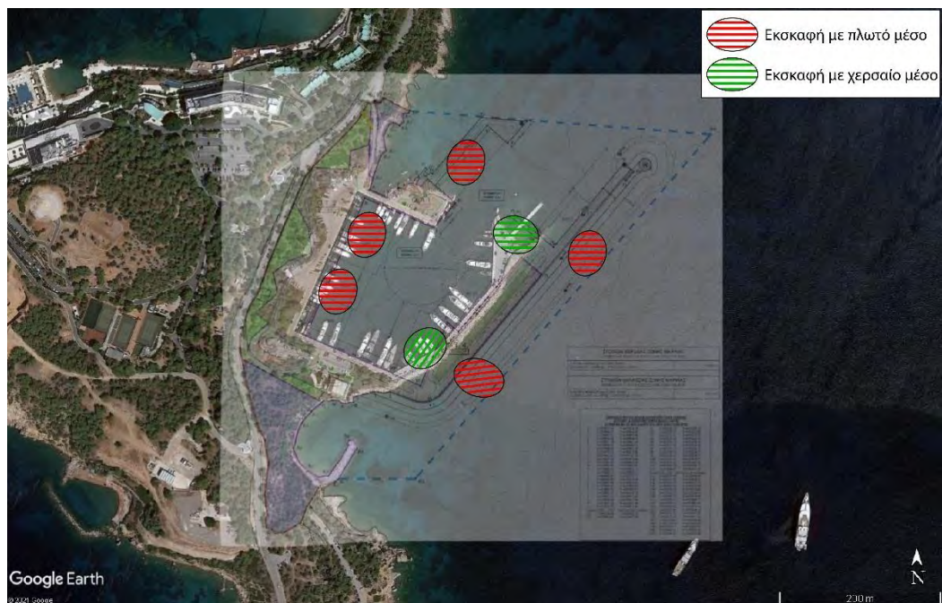
Εικόνα 4: Ενεργές εκσκαφές/βυθοκορήσεις στην περιοχή των έργων της Μαρίνας Βουλιαγμένης κατά τη διάρκεια της 14 ης Σεπτεμβρίου 2021.
