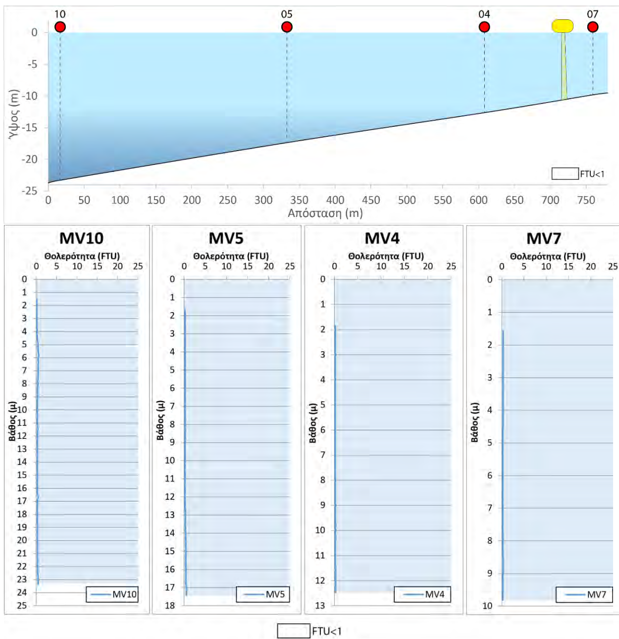
Εικόνα 6: Σχηματική αναπαράσταση της διασποράς/διάχυσης του παραγόμενου νεφελώματος από τις εργασίες εκσκαφής/βυθοκόρησης της 21 ης Σεπτεμβρίου. Για τις θέσεις των μετρήσεων βλέπε την Εικόνα 3.
