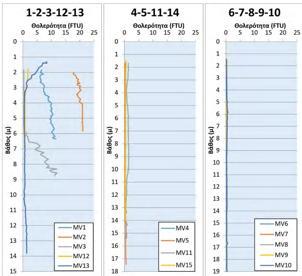
Εικόνα 5: Κατακόρυφες καταγραφές της θολερότητας (σε FTU) στην περιοχή του έργου της Μαρίνας Βουλιαγμένης κατά τη διάρκεια της 21 ης Σεπτεμβρίου 2021. Για τις θέσεις των μετρήσεων βλέπε Εικόνα 3.
