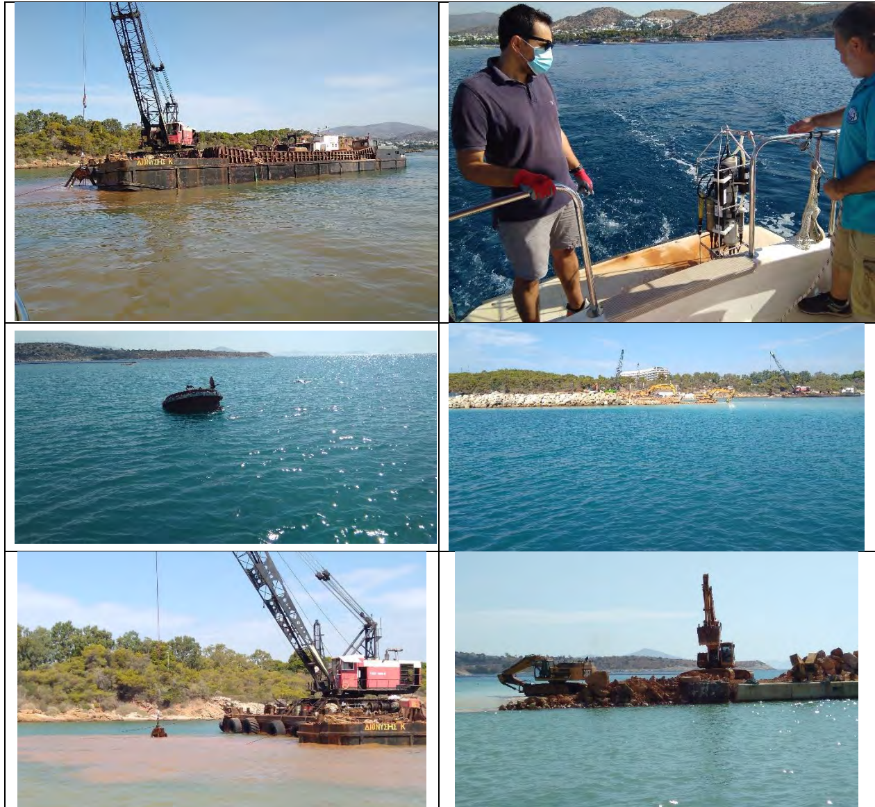
Εικόνα 2: Εργασίες πεδίου με νεφελόμετρο προσαρμοσμένο σε αυτογραφικό σύστημα CTD, το οποίο χρησιμοποιήθηκε για τη συλλογή μετρήσεων στην περιοχή του έργου της Μαρίνας Βουλιαγμένης την 21 η Σεπτεμβρίου 2021
