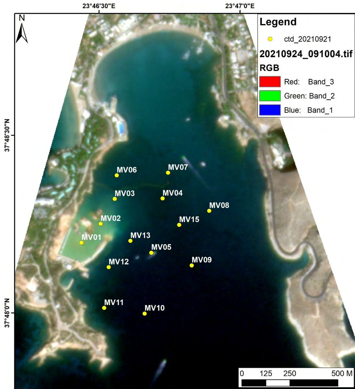
Εικόνα 7: Δορυφορική εικόνα της περιοχής του έργου της Μαρinas Βουλιαγμένης, με τα όρια διασποράς/διάχυσης του επιφανειακού νεφελοειδούς στρώματος (πλουμίου), το οποίο προέκυψε από τις εργασίες βυθοκόρησης της 21 ης Σεπτεμβρίου 2021 (12:10 ώρα Ελλάδος).
