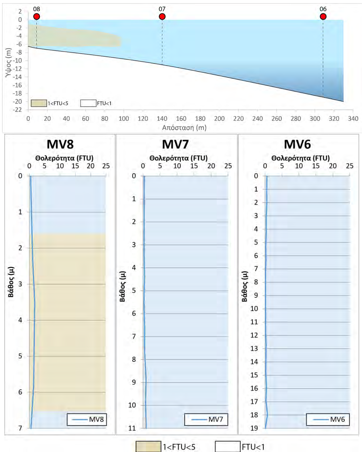
Εικόνα 6: Σχηματική αναπαράσταση της διασποράς/διάχυσης του παραγόμενου νεφελώματος από τις εργασίες εκσκαφής/βυθοκόρησης της 3 ης Νοεμβρίου. Για τις θέσεις των μετρήσεων βλέπε την Εικόνα 3.
