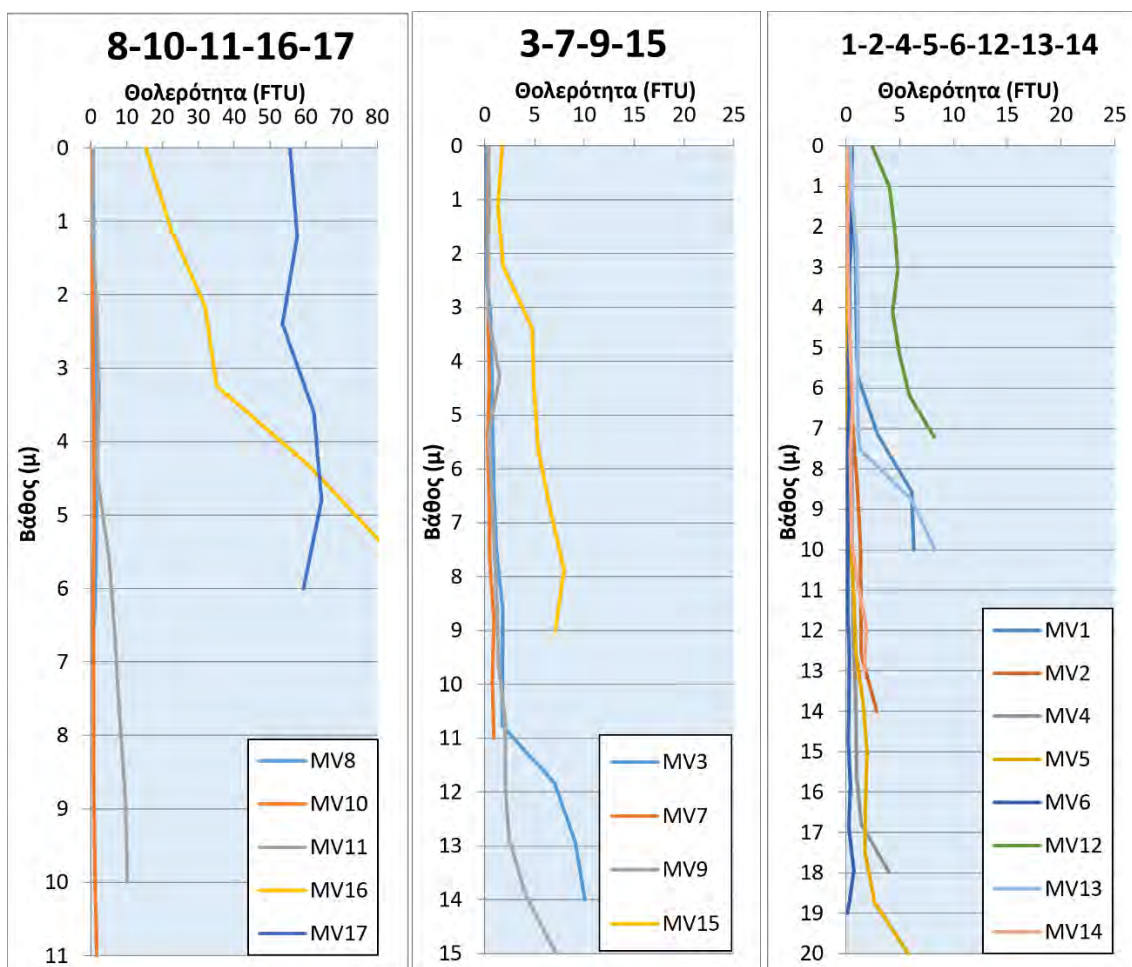
Εικόνα 5: Κατακόρυφες καταγραφές της θολερότητας (σε FTU) στην περιοχή του έργου της Μαρίνας Βουλιαγμένης κατά τη διάρκεια της 3 ης Νοεμβρίου 2021. Για τις θέσεις των μετρήσεων βλέπε Εικόνα 3.
