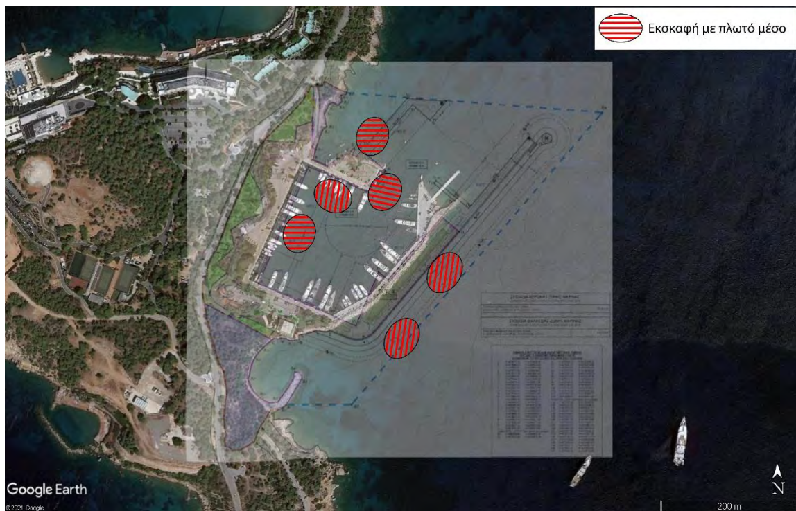
Εικόνα 4: Ενεργές εκσκαφές/βυθοκορήσεις στην περιοχή των έργων της Μαρίνας Βουλιαγμένης κατά τη διάρκεια της 3 ης Νοεμβρίου 2021.
