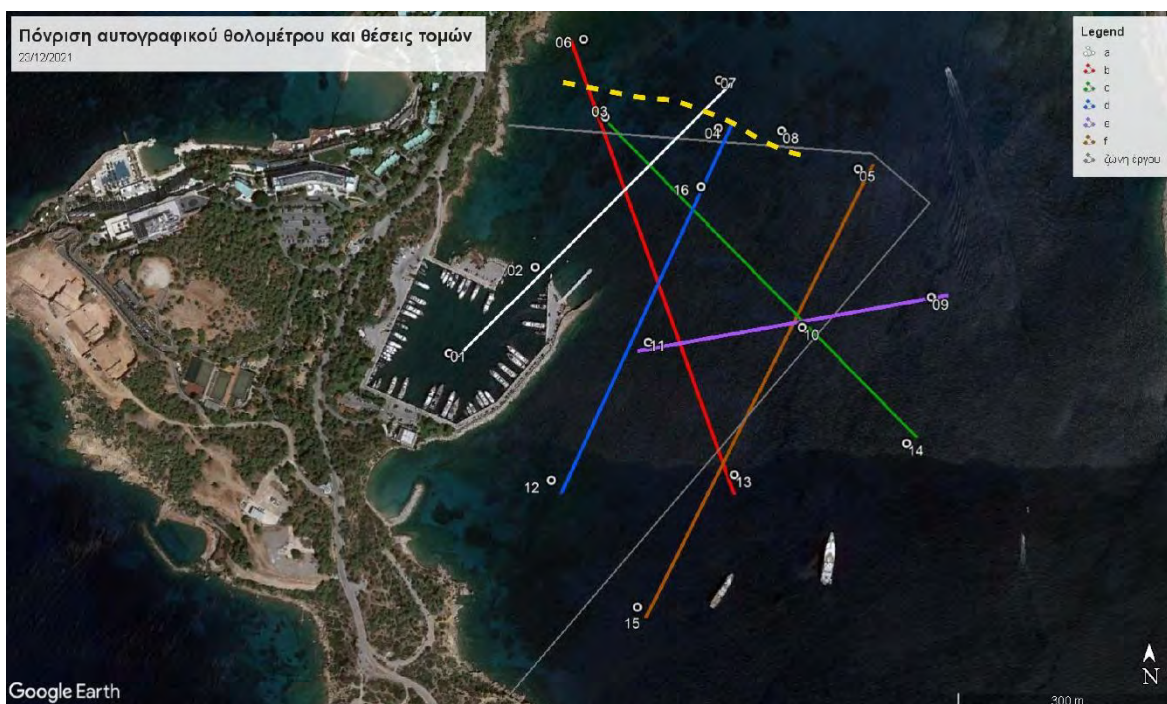
Εικόνα 3: Θέσεις μέτρησης της θολερότητας στην περιοχή του έργου της Μαρίνας Βουλιαγμένης κατά τη διάρκεια της 23 ης Δεκεμβρίου 2021. Η άσπρη, η κόκκινη, η πράσινη, η μπλε, η μωβ και η καφέ γραμμή αντιπροσωπεύουν τις γεωγραφικές θέσεις των τομών των Εικόνων 6α, 6β, 6γ, 6δ, 6ε και 6στ αντίστοιχα. Η διακεκομμένη κίτρινη γραμμή αντιστοιχεί στο τοποθετημένο υδατόφραγμα και η γκρι στα όρια της ζώνης έργου.
