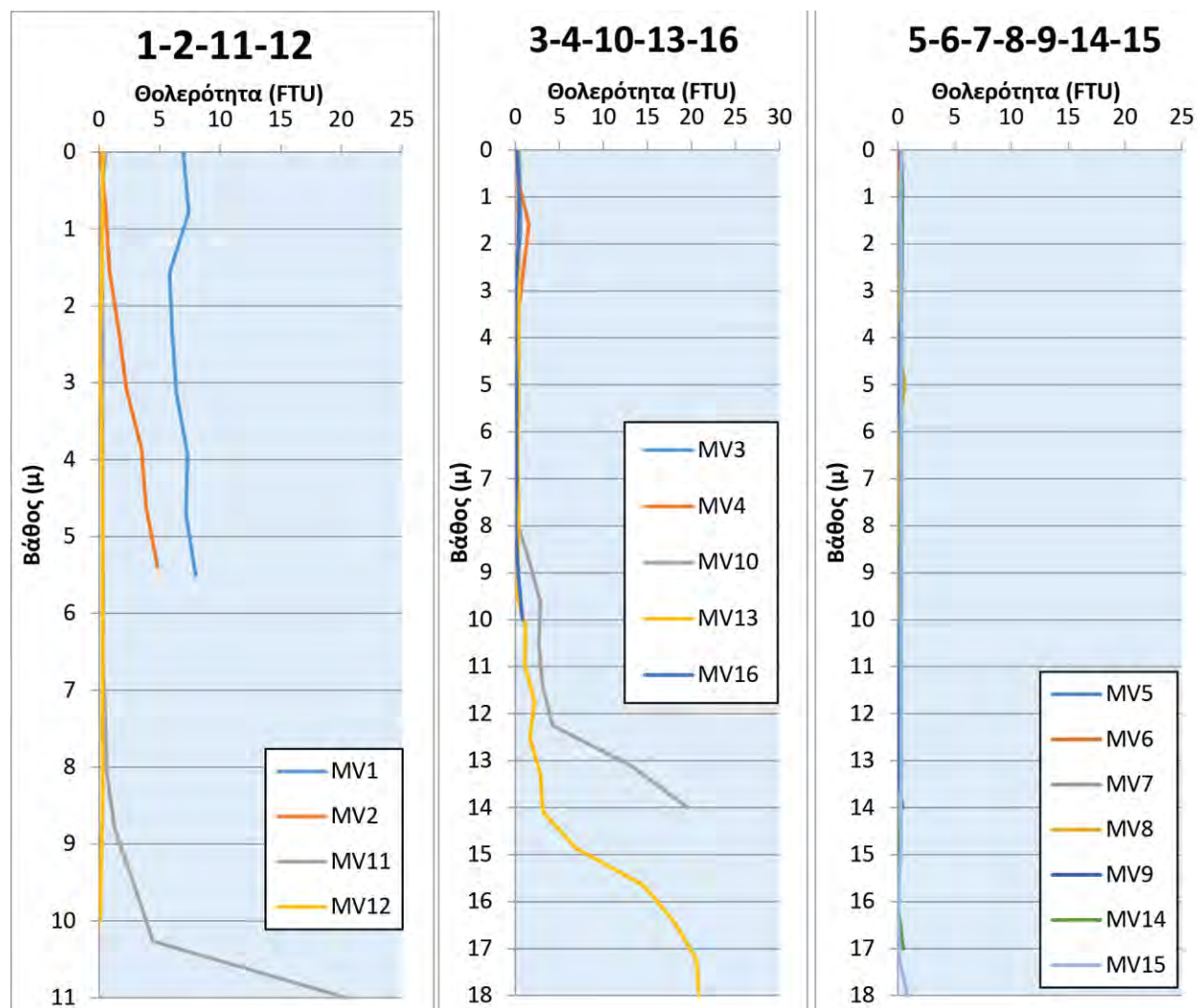
Εικόνα 5: Κατακόρυφες καταγραφές της θολερότητας (σε FTU) στην περιοχή του έργου της Μαρίνας Βουλιαγμένης κατά τη διάρκεια της 23 ης Δεκεμβρίου 2021. Για τις θέσεις των μετρήσεων βλέπε Εικόνα 3.
