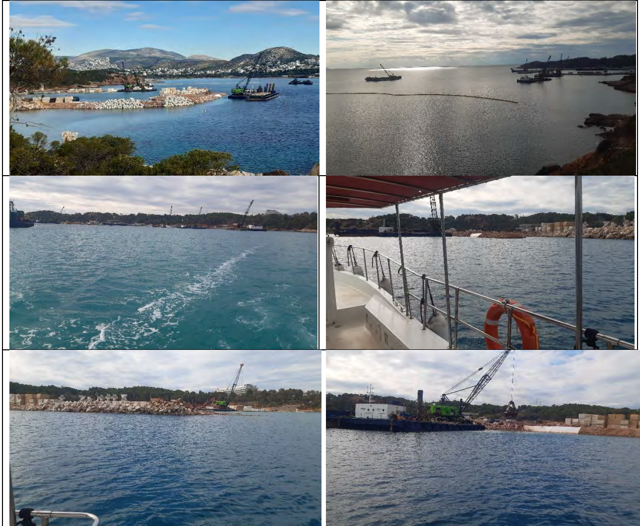
Εικόνα 2: Εργασίες πεδίου με νεφελόμετρο, το οποίο χρησιμοποιήθηκε για τη συλλογή μετρήσεων στην περιοχή του έργου της Μαρίνας Βουλιαγμένης την 23 η Δεκεμβρίου 2021
