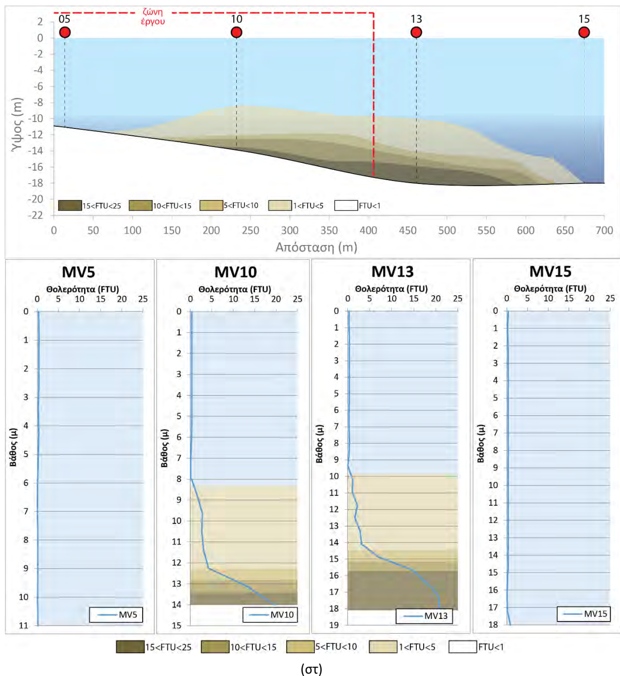
Εικόνα 6: Σχηματική αναπαράσταση της διασποράς/διάχυσης του παραγόμενου νεφελώματος από τις εργασίες εκσκαφής/βυθοκόρησης της 23 ης Δεκεμβρίου. Για τις θέσεις των μετρήσεων βλέπε την Εικόνα 3.
