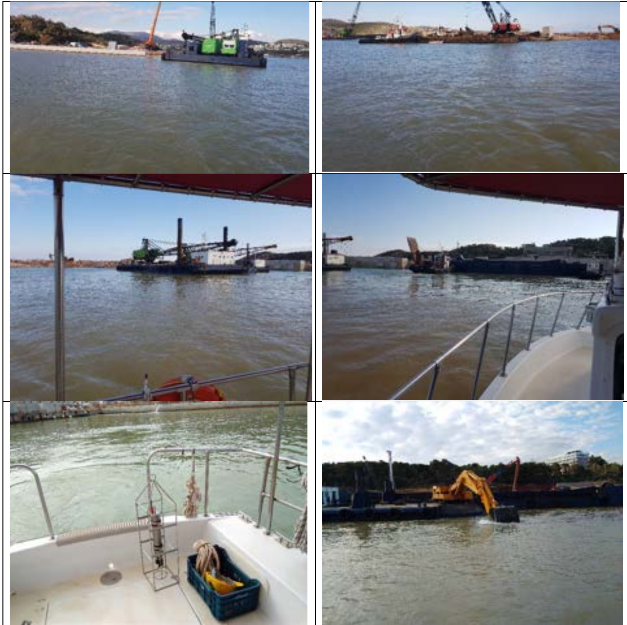
Εικόνα 2: Εργασίες πεδίου με νεφελόμετρο, το οποίο χρησιμοποιήθηκε για τη συλλογή μετρήσεων στην περιοχή του έργου της Μαρίνας Βουλιαγμένης την 4 η Μαρτίου 2022
