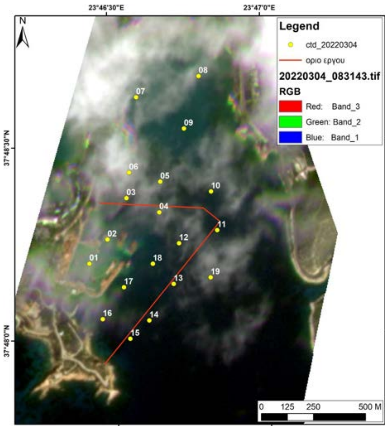
Εικόνα 7: Δορυφορική εικόνα της περιοχής του έργου της Μαρίνας Βουλιαγμένης, με τα όρια διασποράς/διάχυσης του επιφανειακού νεφελοειδούς στρώματος (πλούμιο), το οποίο προέκυψε από τις εργασίες βυθοκόρησης της 4 ης Μαρτίου 2022 (10:31 ώρα Ελλάδας).
