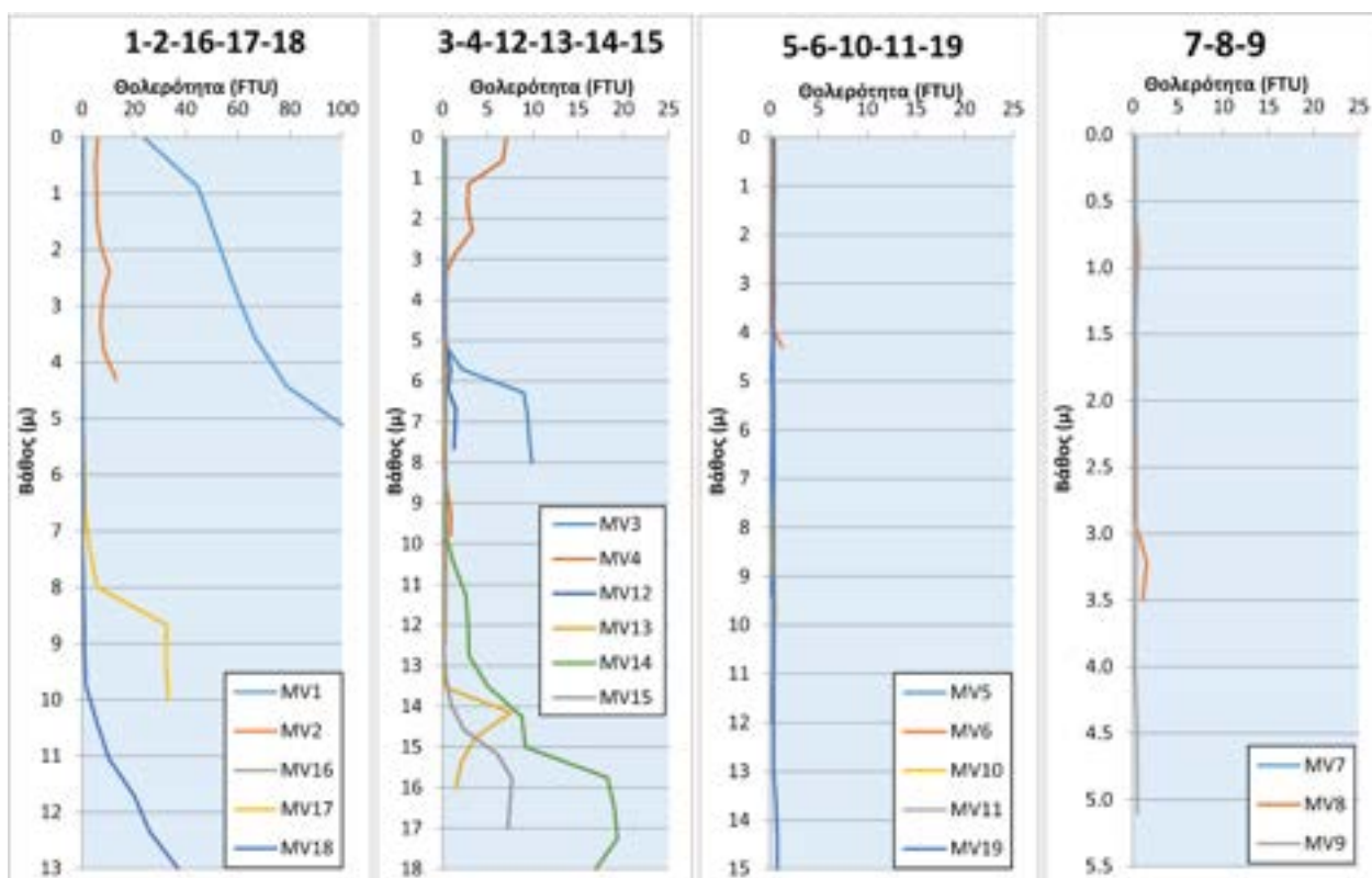
Εικόνα 5: Κατακόρυφες καταγραφές της θολερότητας (σε FTU) στην περιοχή του έργου της Μαρίνας Βουλιαγμένης κατά τη διάρκεια της 4 ης Μαρτίου 2022. Για τις θέσεις των μετρήσεων βλέπε Εικόνα 3.
