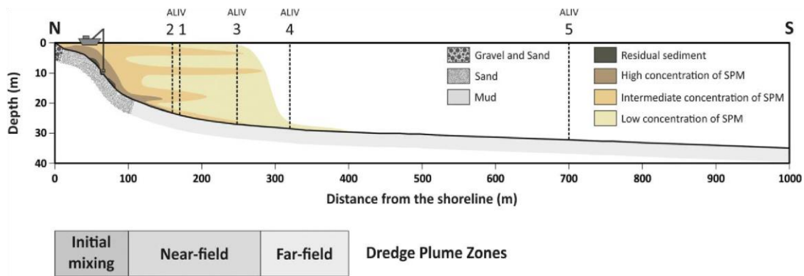
Εικόνα 1: Ζώνες διάχυσης του νέφους των επαναιωρημένων στερεών υλικών που προέκυψε από εντατική βυθοκόρηση στη περιοχή του Αλιβερίου, Νότιος Ευβοϊκός Κόλπος (Kanelloroulos et al. 2020).
