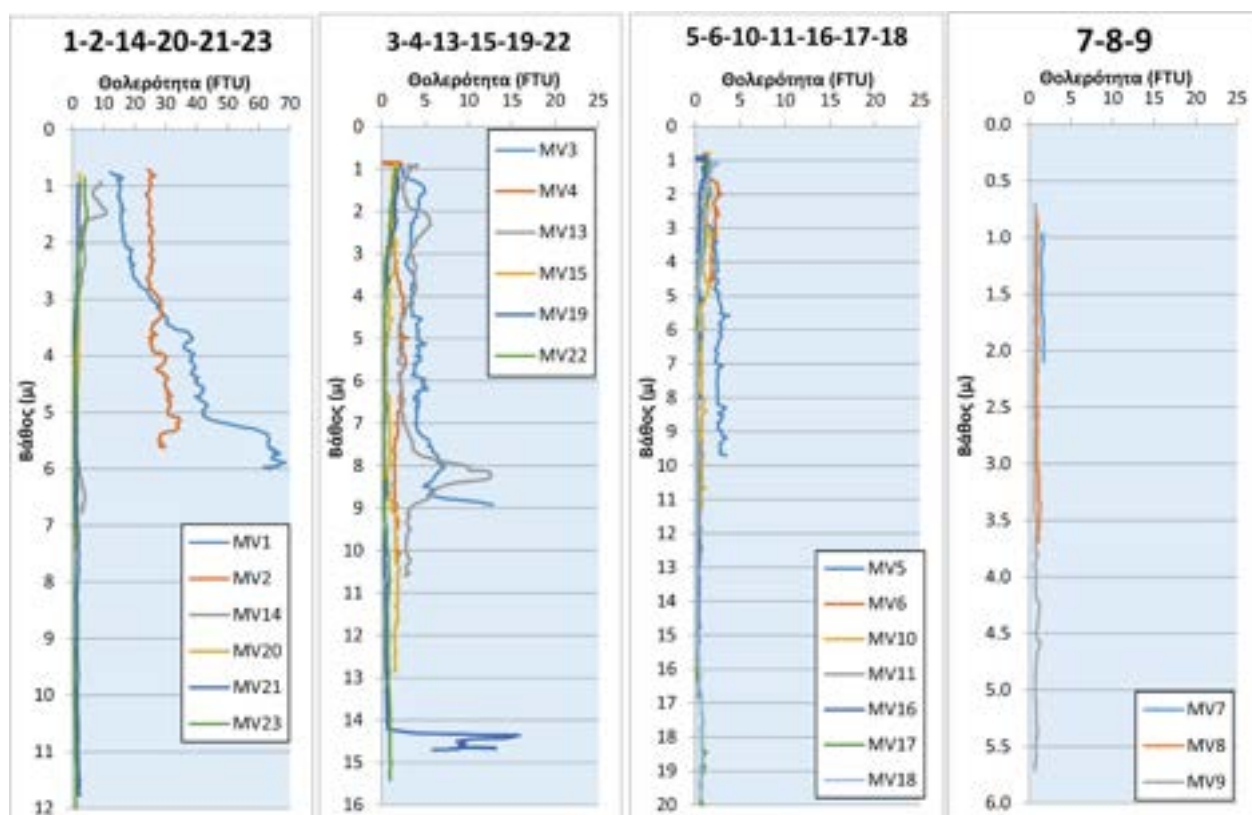
Εικόνα 5: Κατακόρυφες καταγραφές της θολερότητας (σε FTU) στην περιοχή του έργου της Μαρίνας Βουλιαγμένης κατά τη διάρκεια της 20 ης Απριλίου 2022. Για τις θέσεις των μετρήσεων βλέπε Εικόνα 3.
