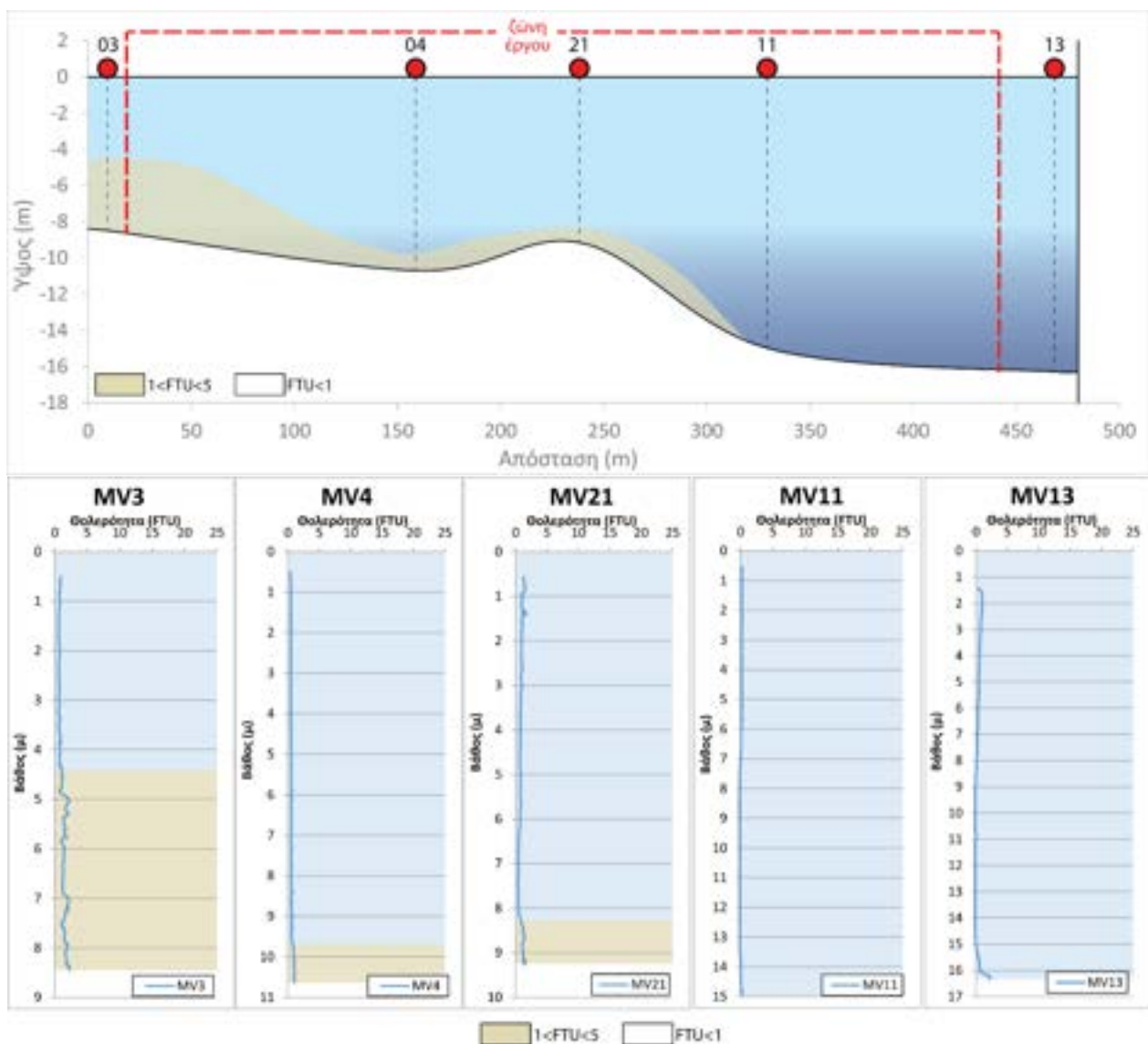
Εικόνα 6: Σχηματική αναπαράσταση της διασποράς/διάχυσης του παραγόμενου νεφελώματος από τις εργασίες εκσκαφής/βυθοκόρησης της 30 ης Ιουνίου 2022. Για τις θέσεις των μετρήσεων βλέπε την Εικόνα 3.
