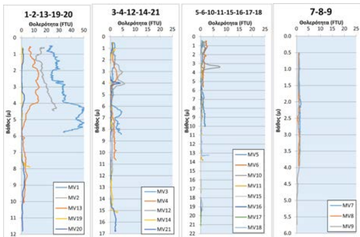
Εικόνα 5: Κατακόρυφες καταγραφές της θολερότητας (σε FTU) στην περιοχή του έργου της Μαρίνας Βουλιαγμένης κατά τη διάρκεια της 30ης Ιουνίου 2022. Για τις θέσεις των μετρήσεων βλέπε Εικόνα 3.
