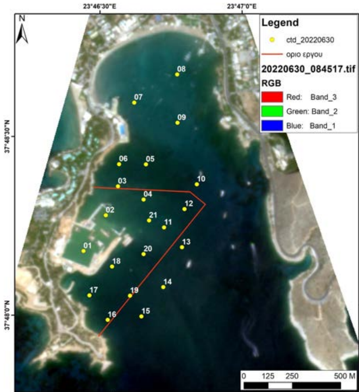
Εικόνα 7: Δορυφορική εικόνα της περιοχής του έργου της Μαρίνας Βουλαγμένης, με τα όρια διασποράς/διάχυσης του επιφανειακού νεφελοειδούς στρώματος (πλουμίου), το οποίο προέκυψε από τις εργασίες βυθοκόρησης της 30ης Ιουνίου 2022 (10:45 ώρα Ελλάδας).
