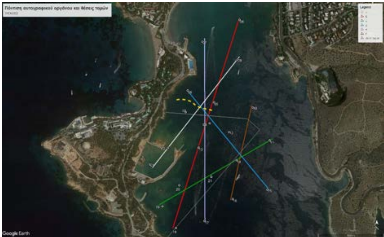
Εικόνα 3: Θέσεις μέτρησης της θολερότητας στην περιοχή του έργου της Μαρίνας Βουλιαγμένης κατά τη διάρκεια της 30ης Ιουνίου 2022. Η άσπρη, η κόκκινη, η πράσινη, η μπλε η μωβ και η καφέ γραμμή αντιπροσωπεύουν τις γεωγραφικές θέσεις των τομών των Εικόνων 6α, 6β, 6γ, 6δ 6ε και 6στ, αντίστοιχα.
